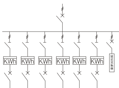
图1 接线图
