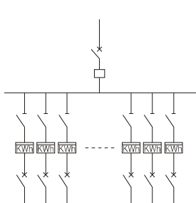
图1 接线图
