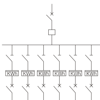
图1 接线图
