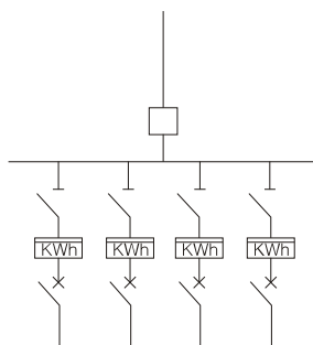
图1 接线图
