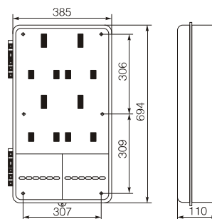
图2 外形及安装尺寸
