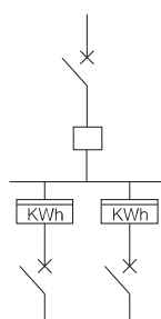
图1 接线图
