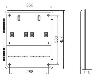
图2 外形及安装尺寸
